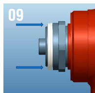
9.- Acabar de introducir manualmente la junta en la ranura
