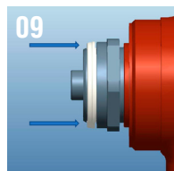
9.- Termine a inserção manual da junta na ranhura
