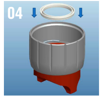
4.- 將唇形密封圈放置在指示位置
